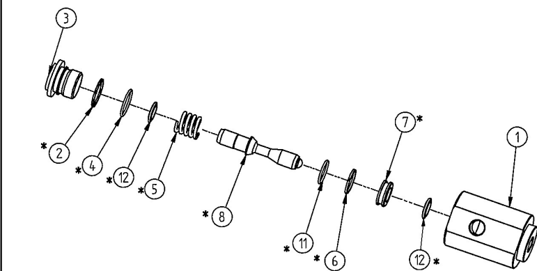
⑦バルブASSY
